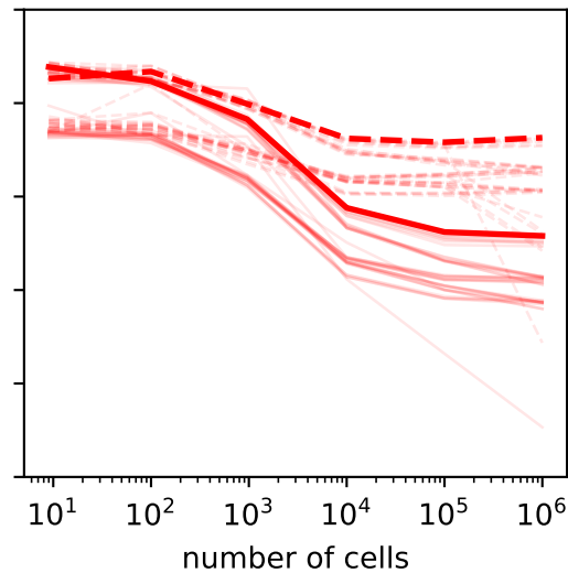
(e) trilinos
