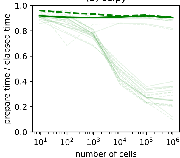
(b) scipy
