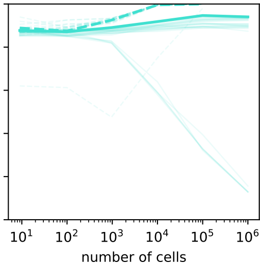
(d) petsc 3.20.2
