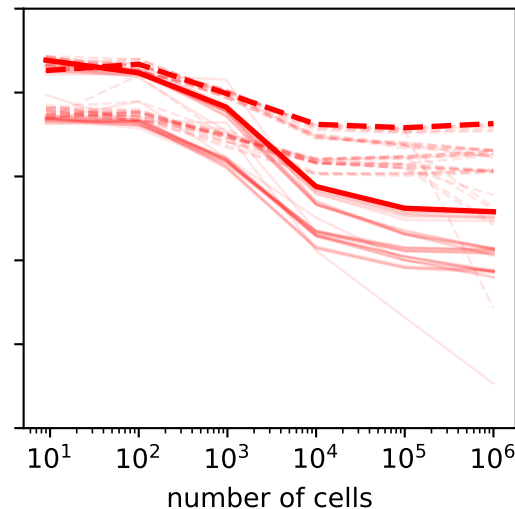
(e) trilinos
