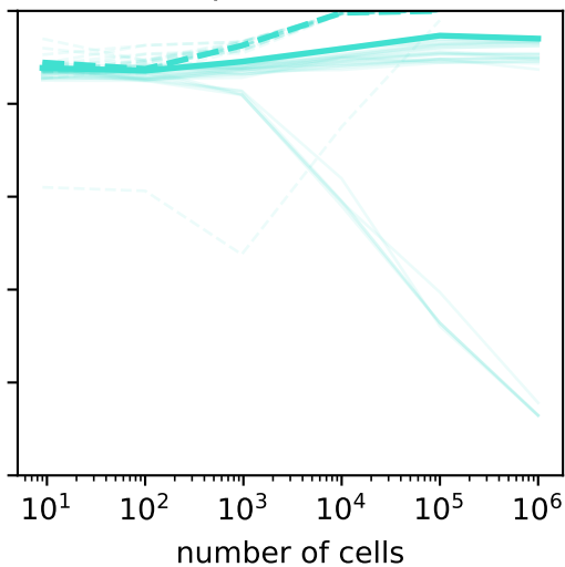
(d) petsc 3.20.2
