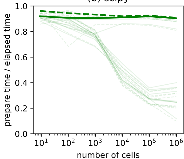
(b) scipy
