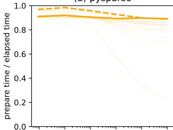
(a) pysparse
